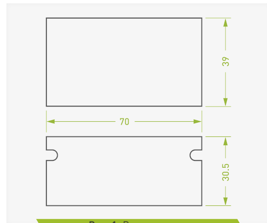
Рис. 1. Размеры модуля
