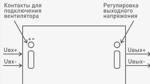
Рис. 2. Схема подключения
