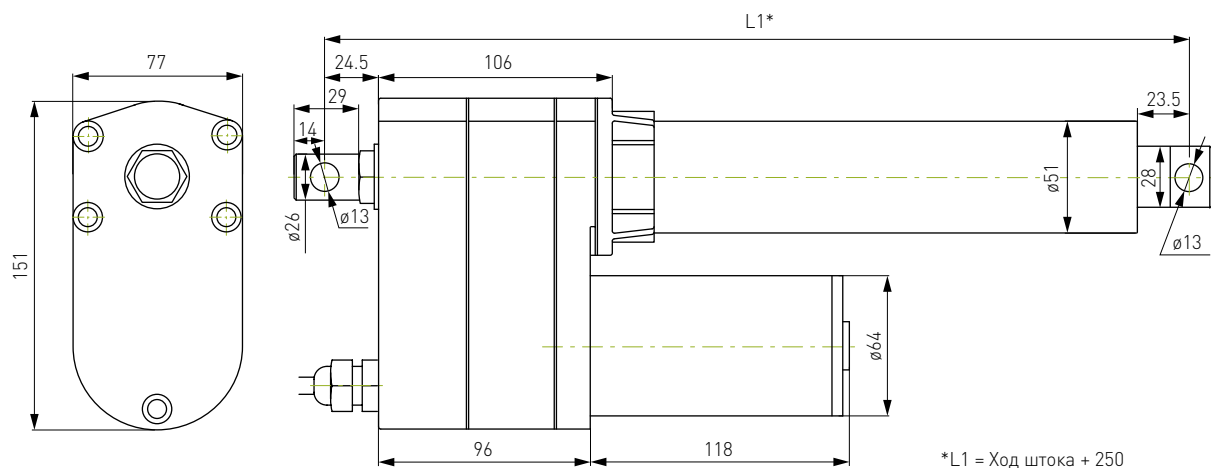
Рисунок 1 – Габаритные и присоединительные размеры (мм) актуаторов TGC.
