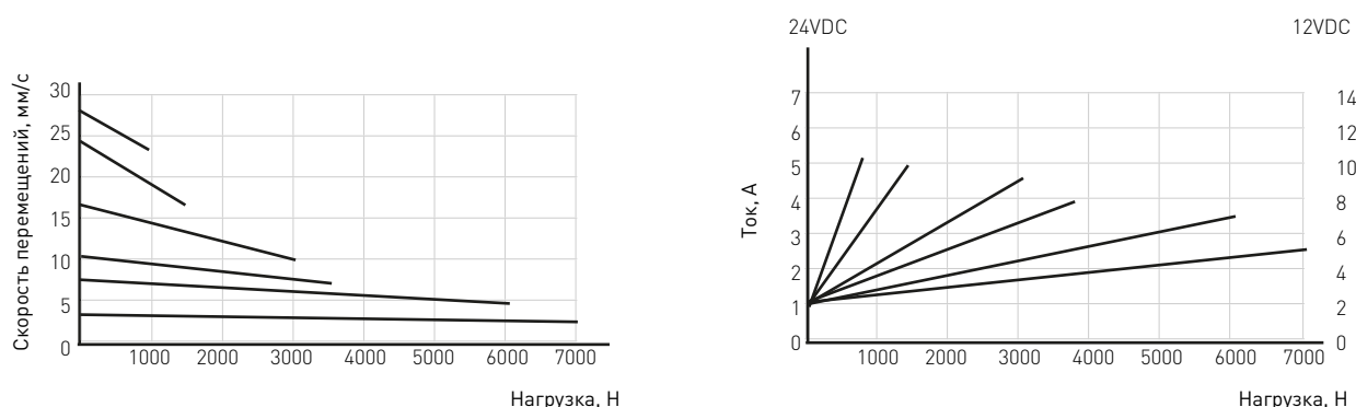
Рисунок 2 – Результаты испытаний, полученные при работе двигателя 24VDC.
