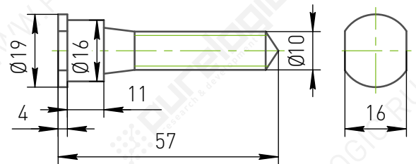
Винт крепления - КР125
