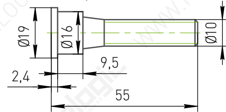
Винт крепления - КР96
